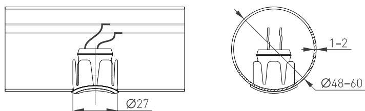
Рис. 2. Установка светильника
