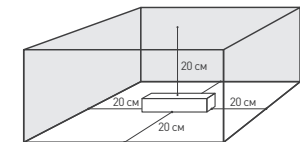
Рис. 3. Свободное пространство вокруг источника
