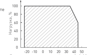
Рис. 4. Максимальная допустимая нагрузка, % от мощности источника
