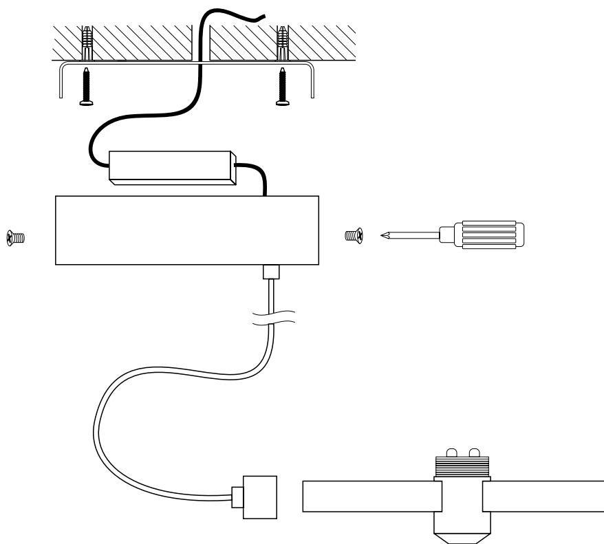
Рис. 2. Установка потолочного короба на поверхность и шинопровод
